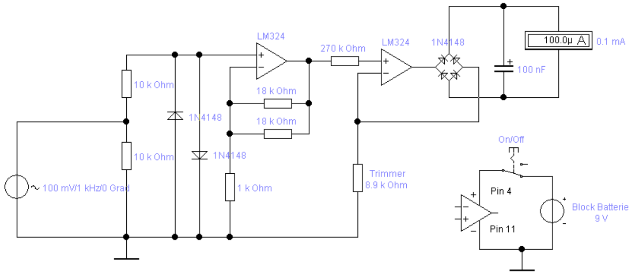
AC - Millivoltmeter von 1 - 100 mV bei 1 KHz Fehler <1%
